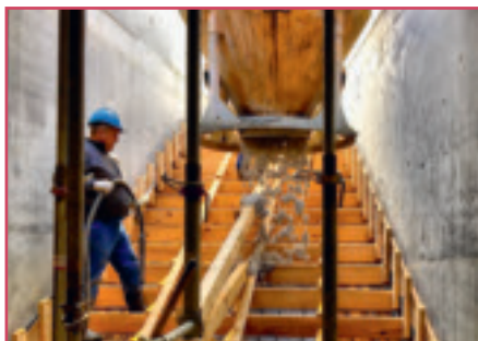
Gros plan sur le bétonnage de l'escalier qui mènera le public au foyer du Théâtre
